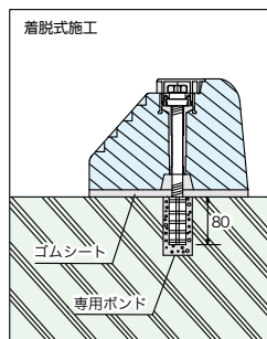
アスファルト舗装用 アンカーピン 120用
