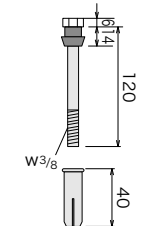
コンクリート舗装用 アンカーピン 120用
