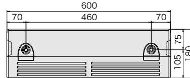
NSP-120(G)B 参考重量 25kg
