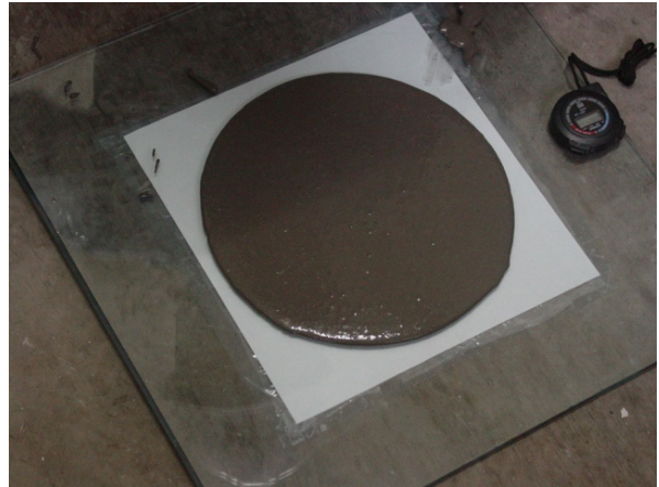
フロー試験
