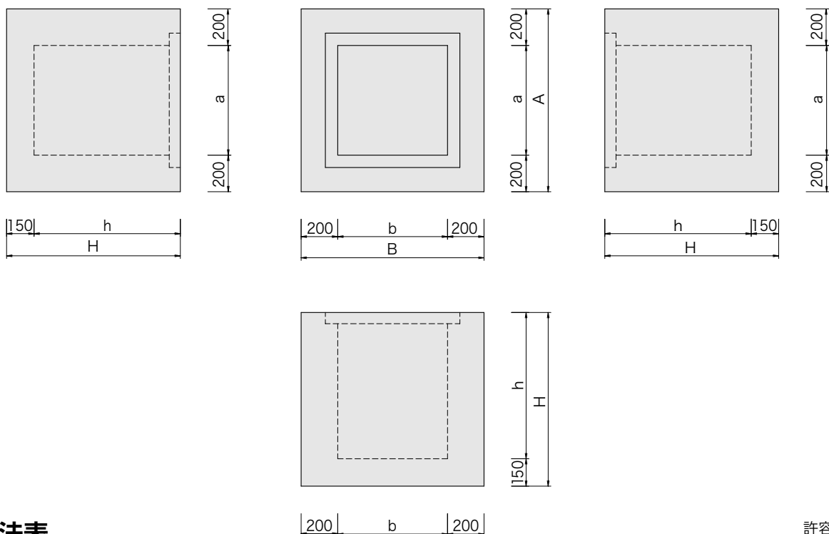
寸法表
